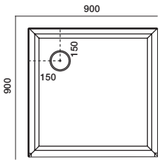
900x900 LH or RH
