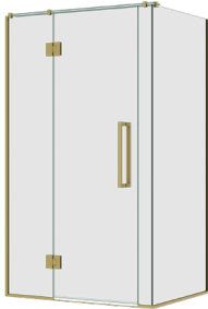
1200 Door Set 1200Wx900Dx1950H
