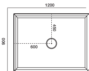
1200x900 LH or RH
